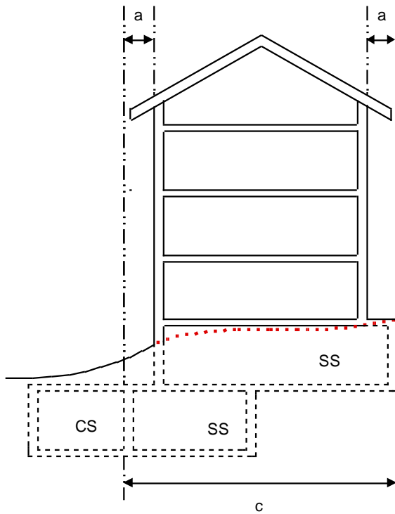
Figure 6.2 Sous-sols
