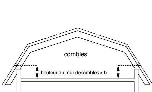
petite hauteur du mur de combles admise grande hauteur du mur de combles admise
