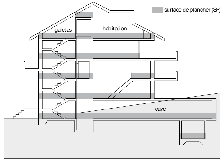
coupe:
