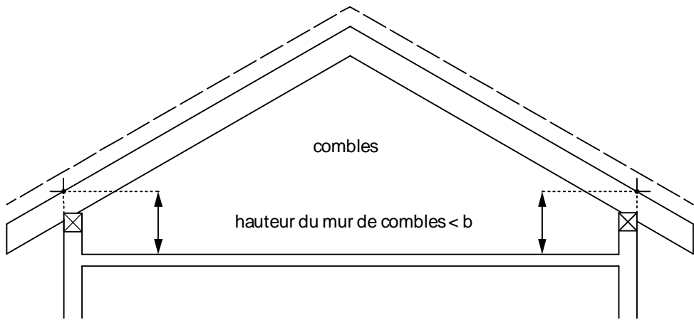
b hauteur du mur de combles admise
