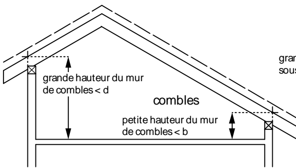
petite hauteur du mur de combles admise grande hauteur du mur de combles admise
