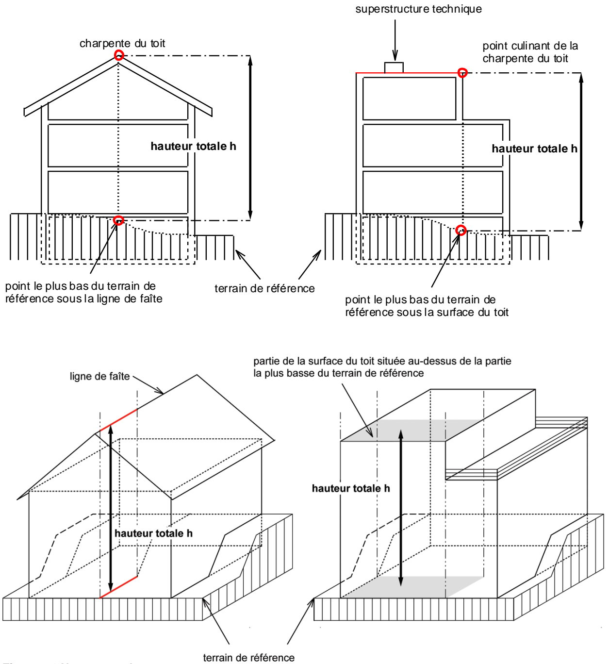
Figure 5.1 Hauteur totale
