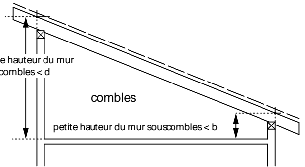
b hauteur du mur de combles admise
