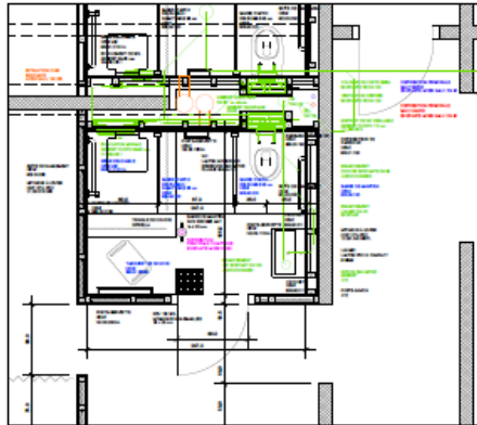
WC/DOUCHE 33 1:20
