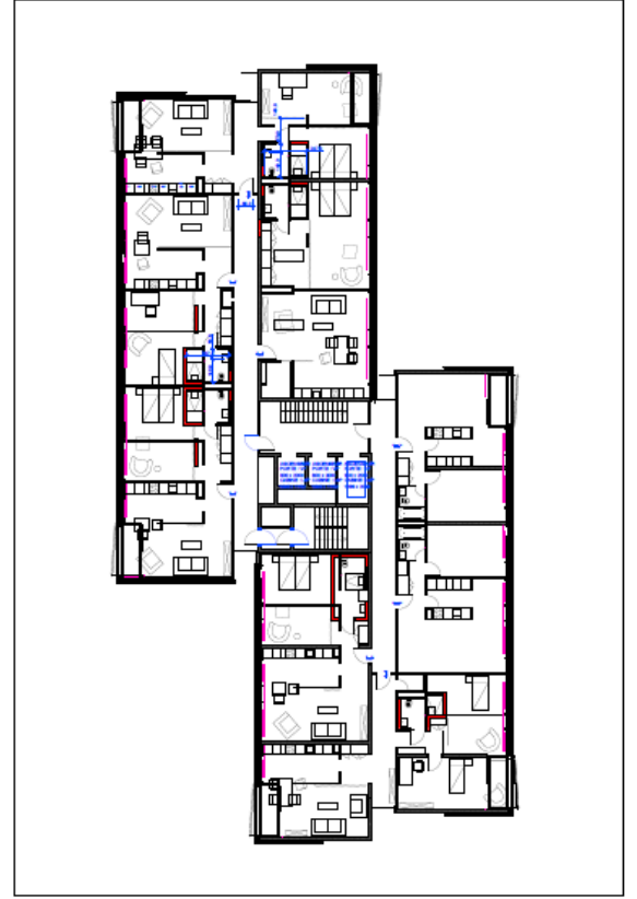
GRUNDRISS 3 - 9.00 1:100
