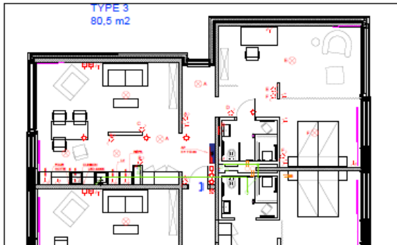
GRUNDRISS 33 1:50
