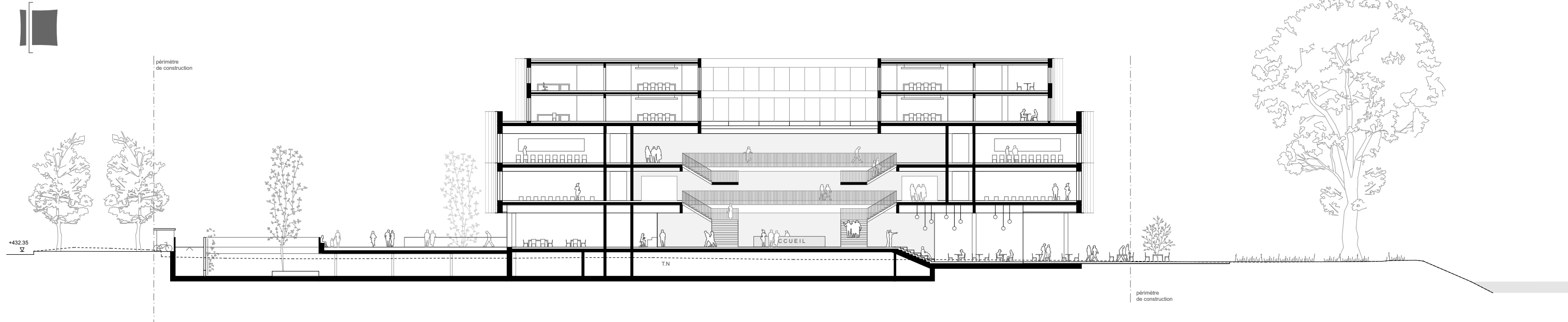
COUPE LONGITUDINALE - HALL D'ENTRÉE 1 : 200
