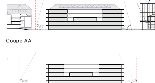
Coupe BB
