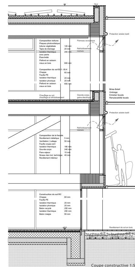
Coupe constructive 1:50
