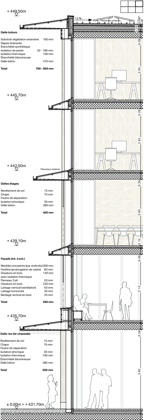
Coupe constructive 1:50
