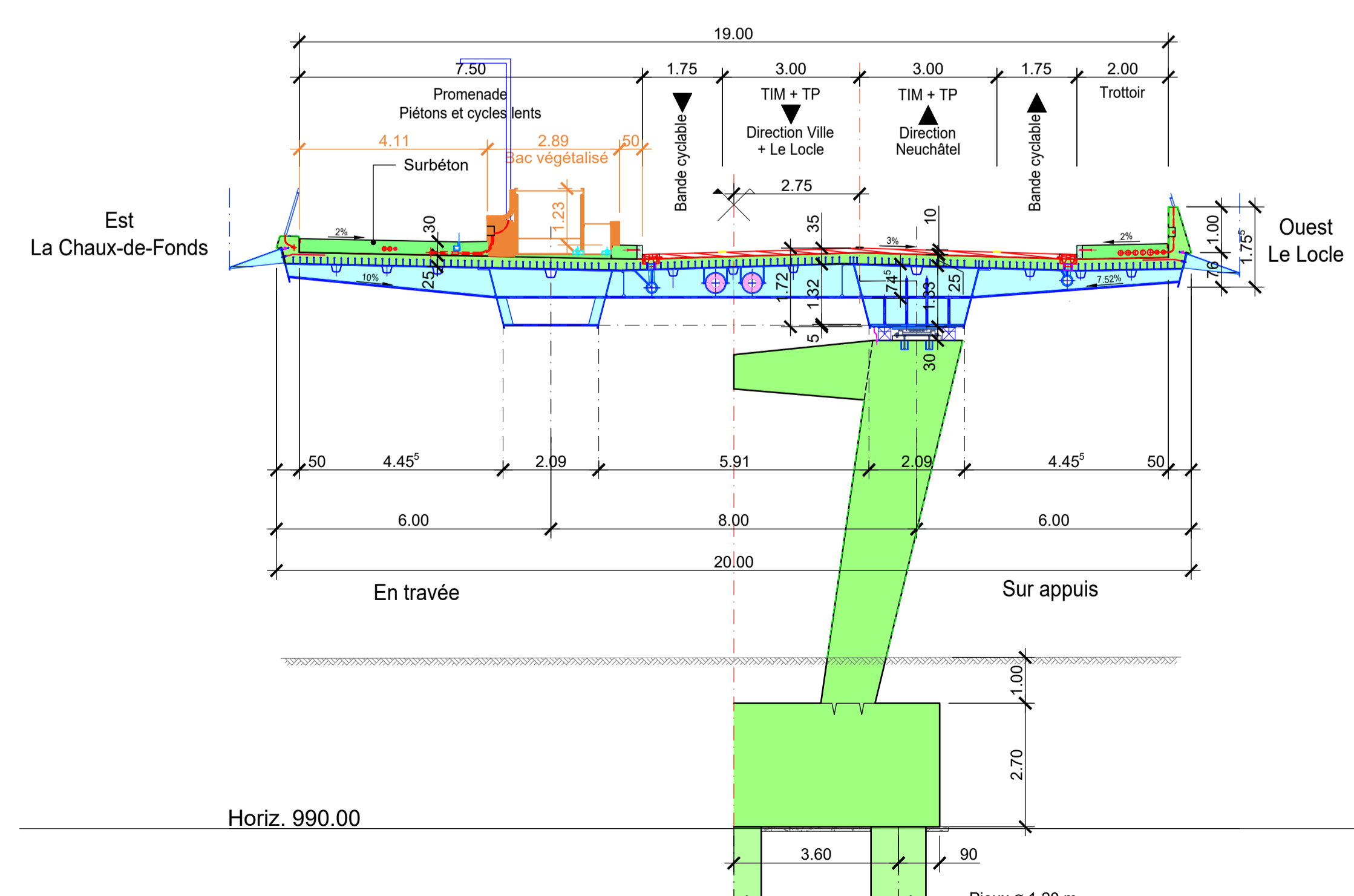
Coupe transversale type 1:100
