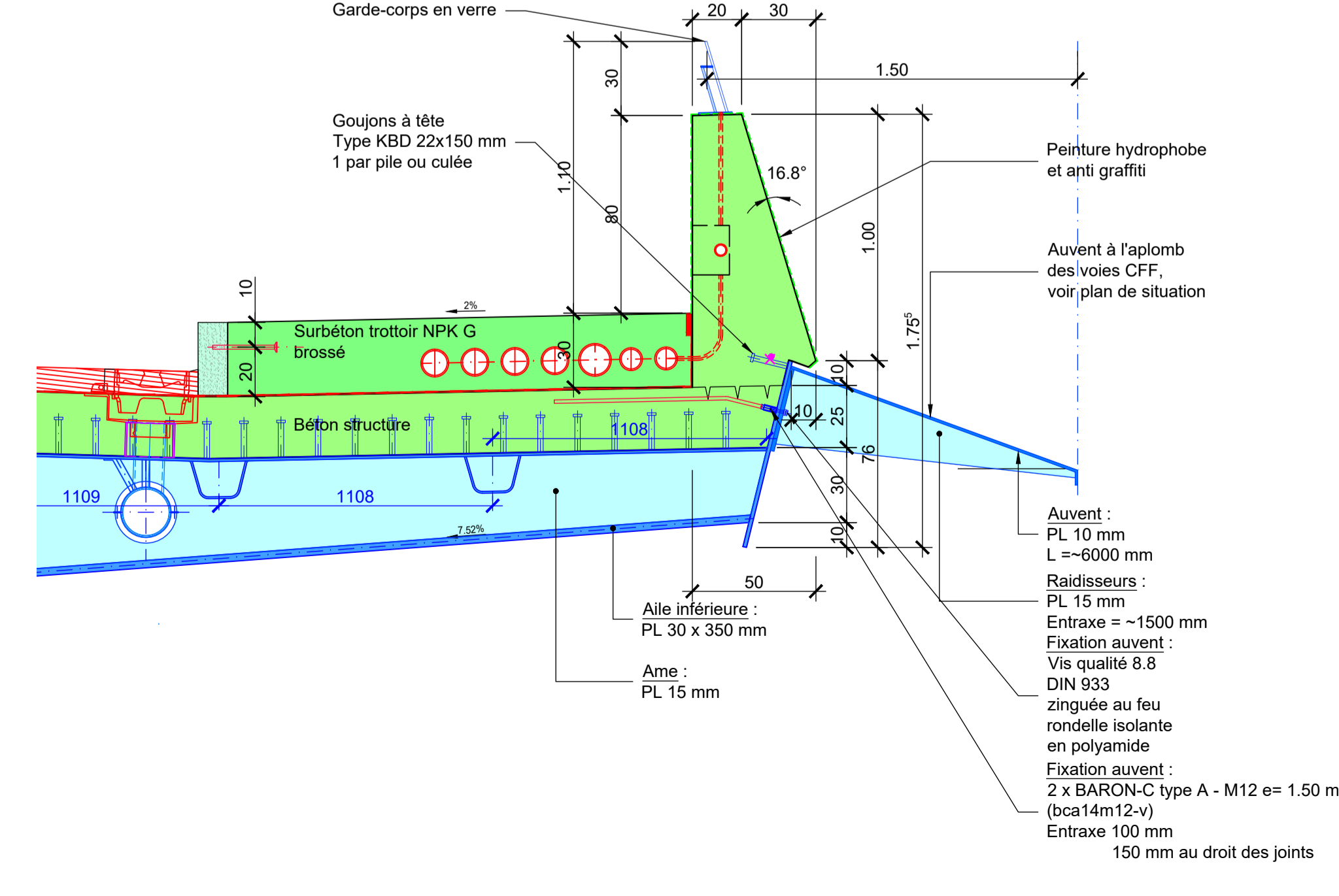
Coupe sur type parapet Ouest 1:20 avec auvent
