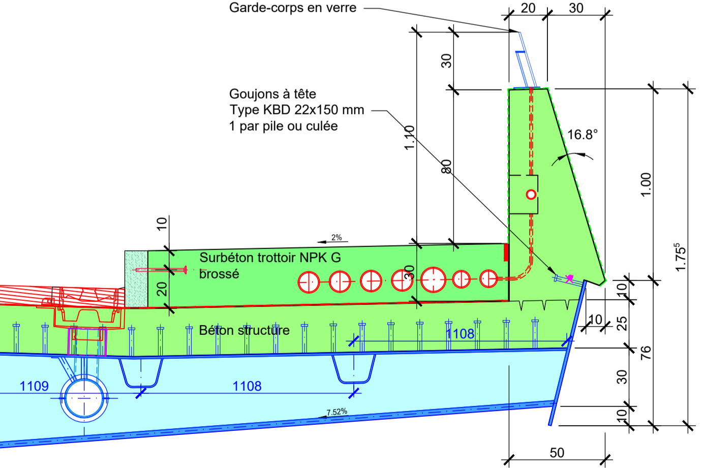
Coupe type sur parapet Ouest 1:20
