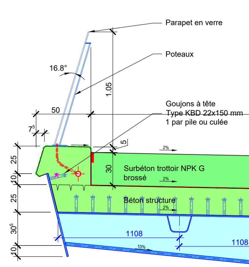
Coupe type sur parapet Est 1:20
