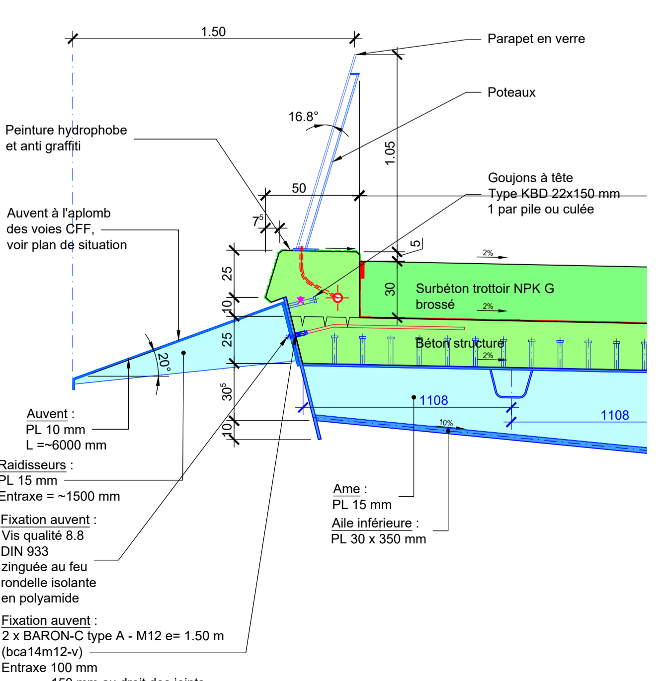
Coupe type sur parapet Est 1:20 avec auvent
