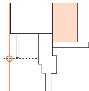
Cadre entre murs en position intérieure, hauteur de niche 35 cm
